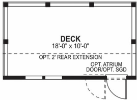
OPTIONAL DECK
